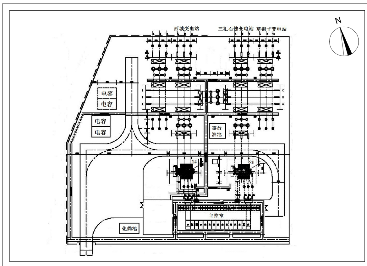
图 4-2 渠县南阳庆丰 110kV 输变电工程南阳庆丰变电站平面布置图
